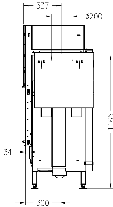
Seitenansicht M~1:20
